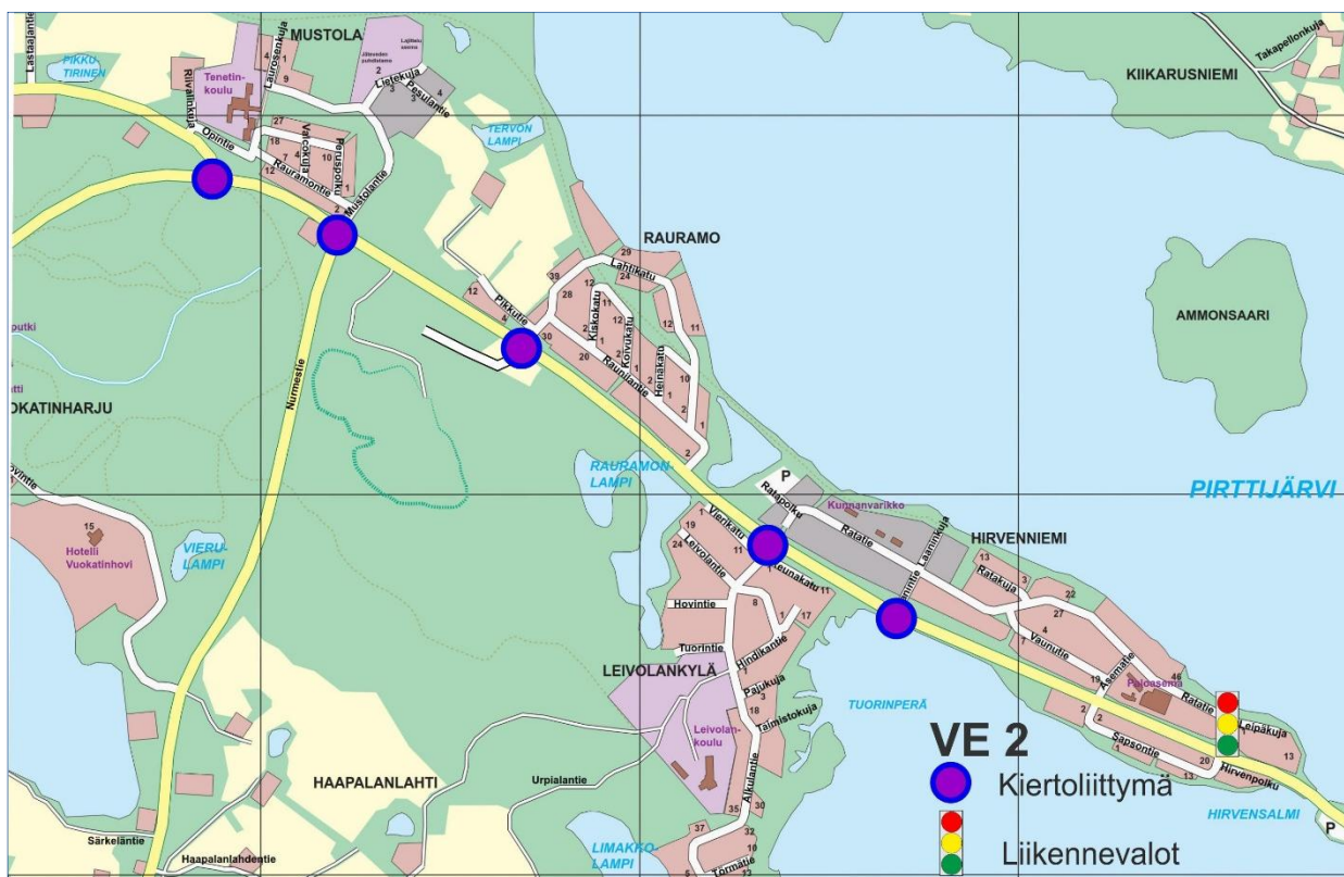
Kuva 31. Pohjavaarantien ja Hirvensalmen välillä olevien pääliittymien kehittämisehdot.
