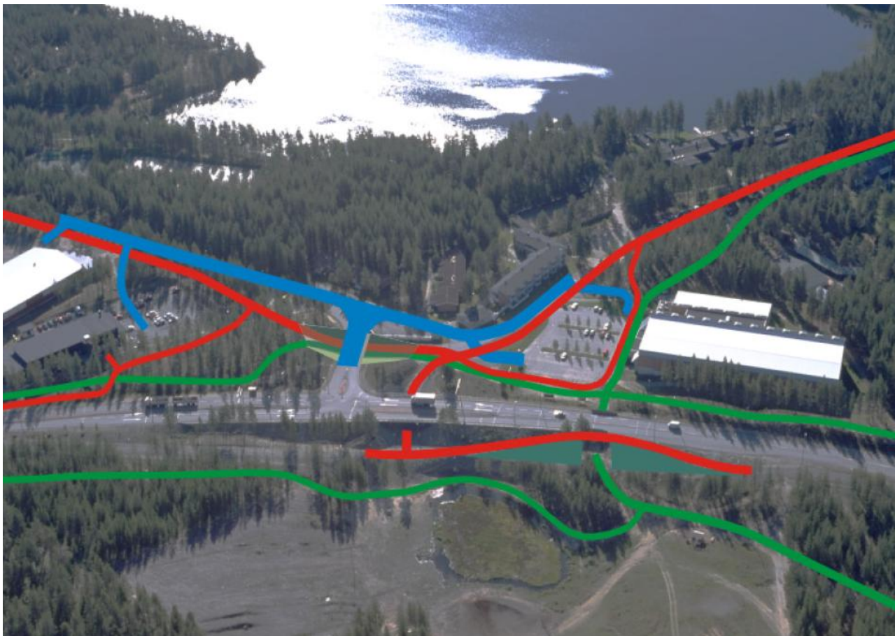
Kuva 24. Vuoden 2000 Vuokatin liikennejärjestelmäsuunnitelmassa esitetyt ratkaisut Urheiluopiston alueen liikennejärjestelyiksi (VE 1).
