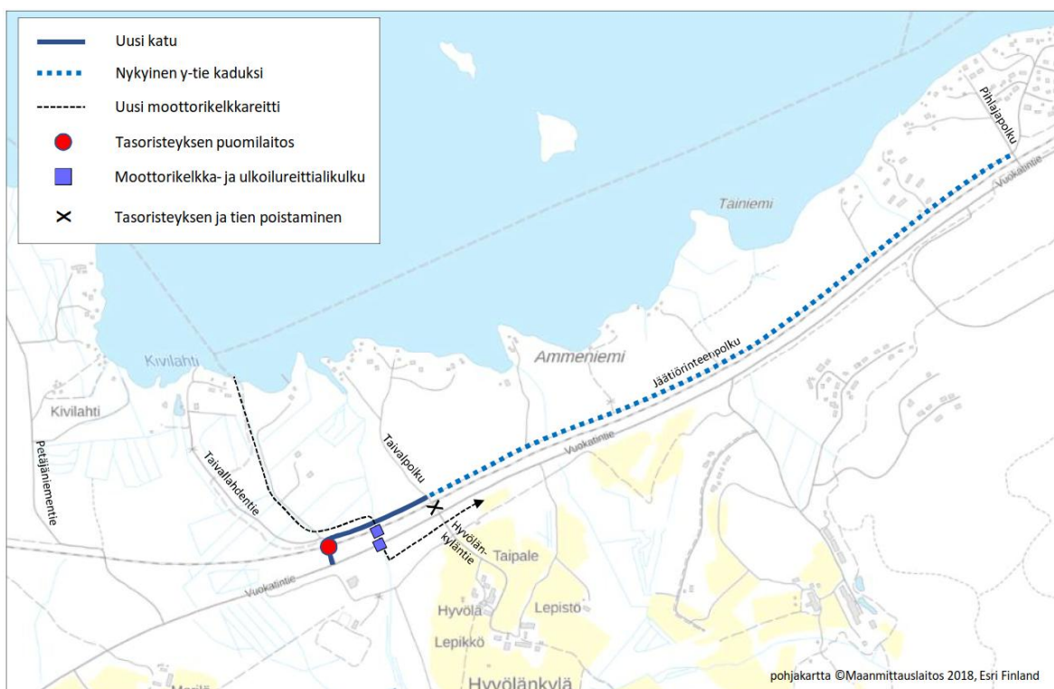
Kuva 35. Kivilahti-Ammenniemen rinnakkaistiejärjestelyt ja moottorikelkkareitin kehittäminen 1.vaiheessa.
