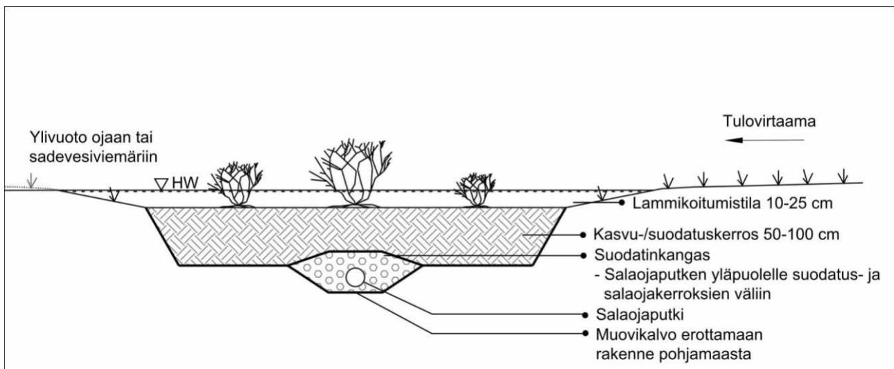
Kuva 22. Tyypin kuva kalvorakenteella eristetystä suodatuspaineesta. (FCG)
