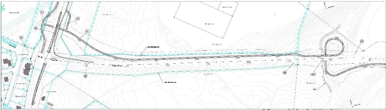
Kuva 21. Nurmetien ja Kainuuntien liittymäratkaisu ja Nurmetien kevyen liikenteen väylä / Sitowise Oy.
