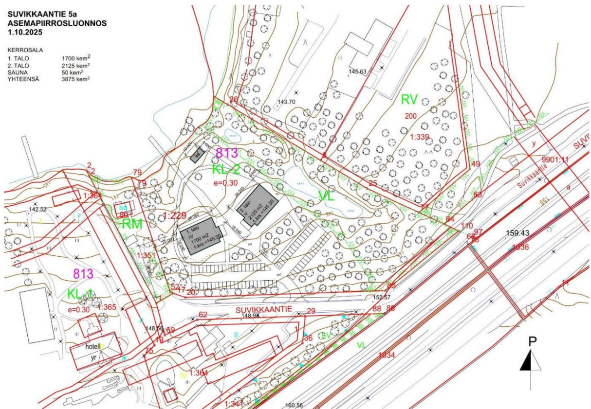
Kuva 1. Suvikkaantie 5a asemapiirrosluonnos
